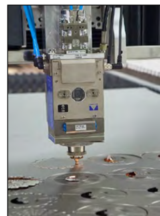
Precitech skærehoved
