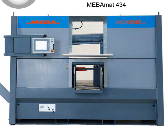
MEBAmat 434
