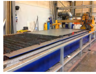
Microstep plasmaskærer Type CPL4501.20, årg. 2002 Kjellberg plasma HI Focus 100
