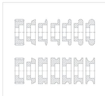
AK 80 standardruller 7 sæt ruller medfølger
