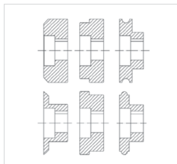
AKM 400 standardruller 3 sæt ruller medfølger
