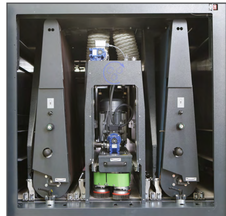
Rulleenhed Ø250 / Tangential børstesystem, Planetarisk system / Elektronisk slibesæt
