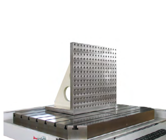
Vinkelblok
