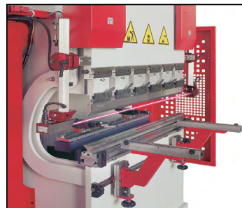
Støttearme foran
